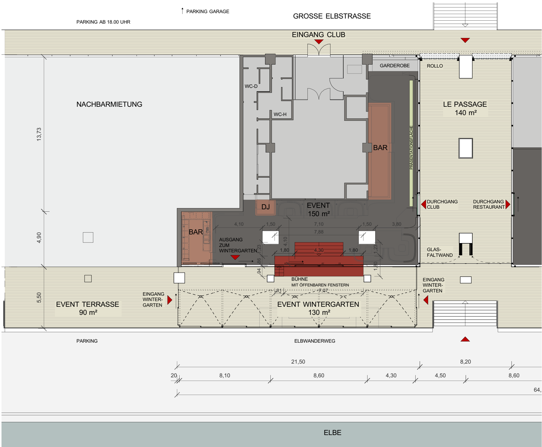
Grundriss M.1:200
